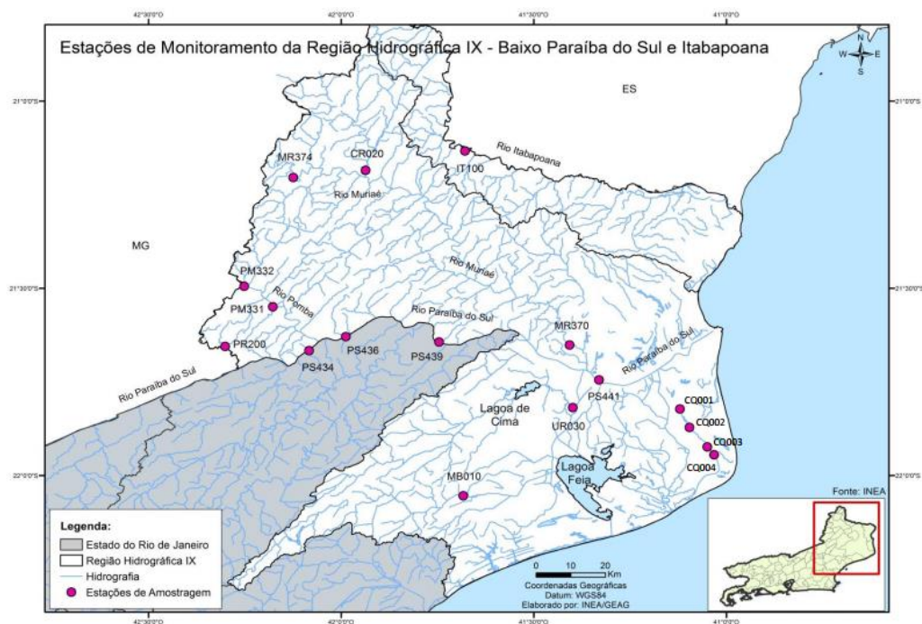
Figura 8. Estações de Amostragem da Região Hidrográfica IX.
