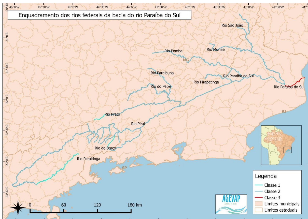
Figura 9. Enquadramento dos rios federais da bacia hidrográfica do rio Paraíba do Sul.
