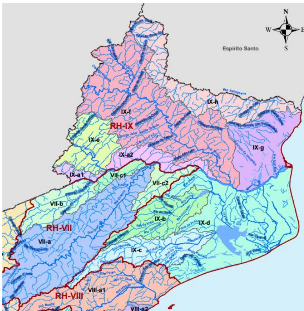
Figura 7. Divisão da RH IX em UHP.
